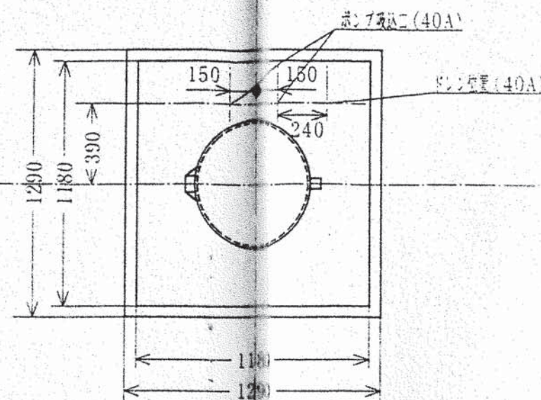
受水槽座部寸法
