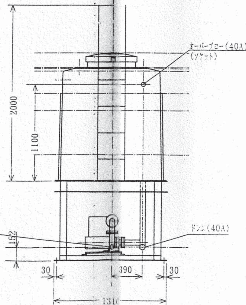
受水槽座部寸法
