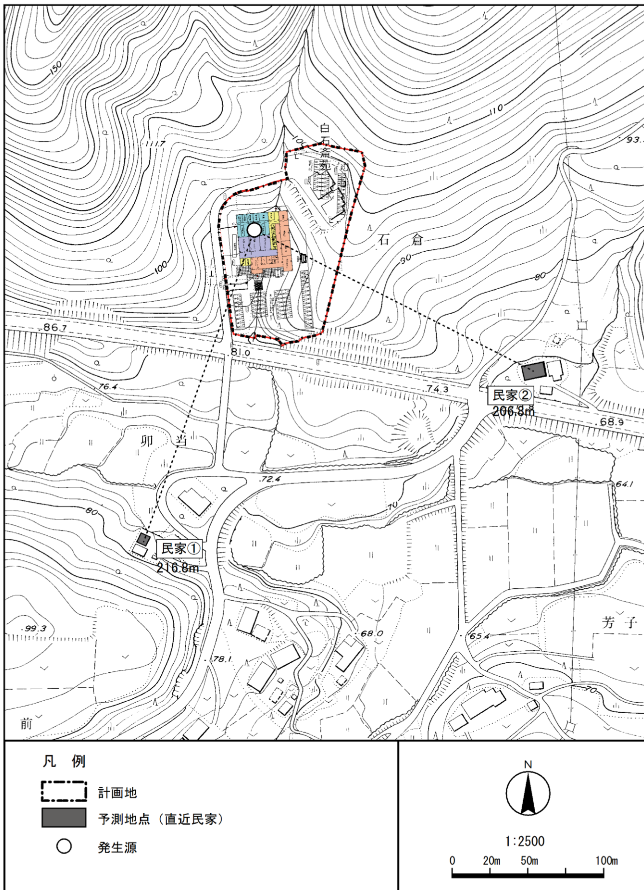
図 5-2-2 設備の配置位置及び振動予測地点
