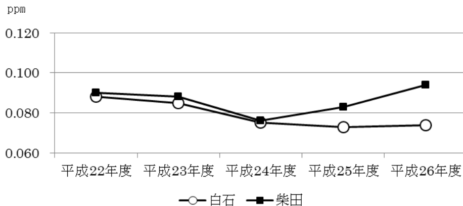
図 3-1-5 光化学オキシダントの経年変化
