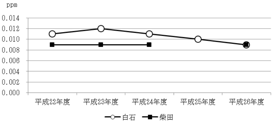
図 3- 1-4 二酸化窒素の経年変化
