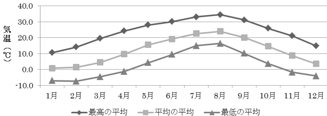
図 2-2-3 白石局における気温の推移
