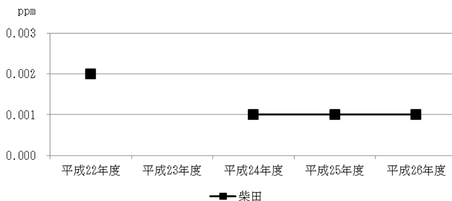
図 3- 1-2 二酸化硫黄の経年変化
