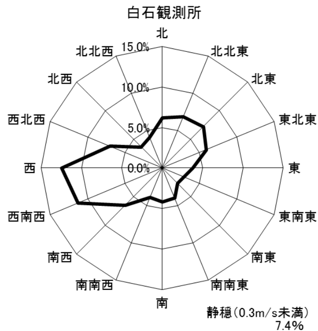
図 2-2-5 白石局における風配図（平成 27 年）
