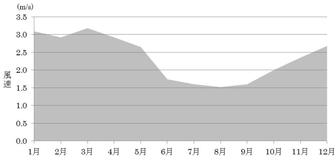
図 2- 2-6 白石局における風速の推移
