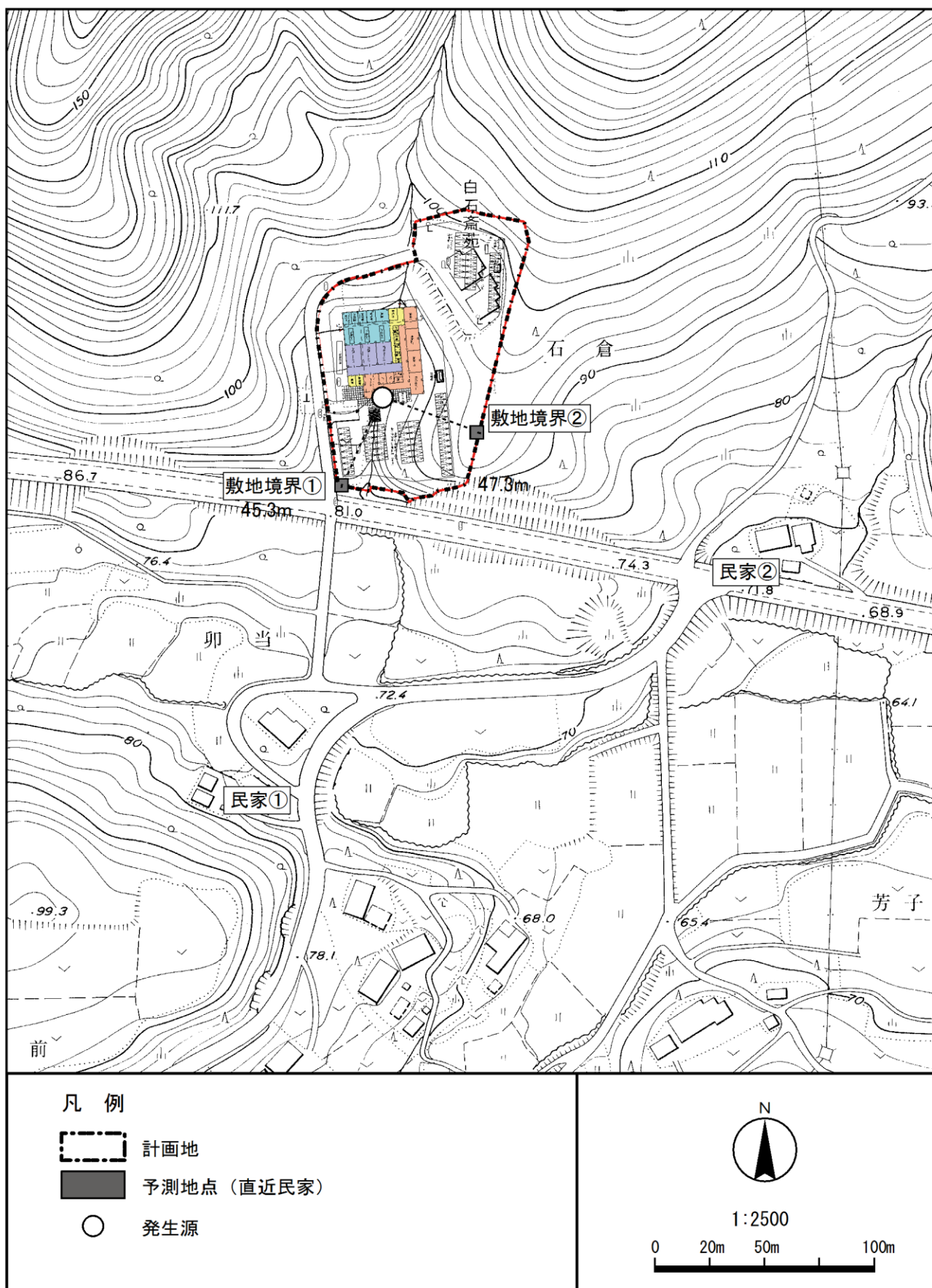
図 5- 2-1 建設機械配置位置及び振動予測定点
