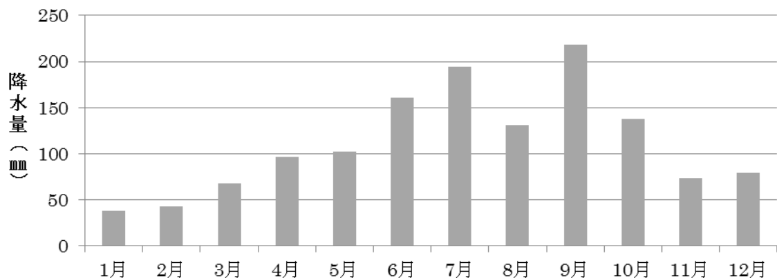
図 2- 2-4 白石局における降水量の推移
