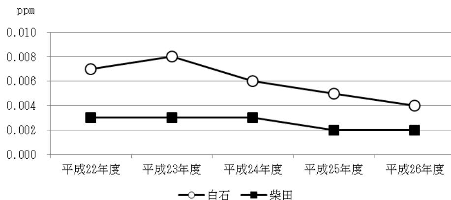
図 3-1-3 一酸化窒素の経年変化
