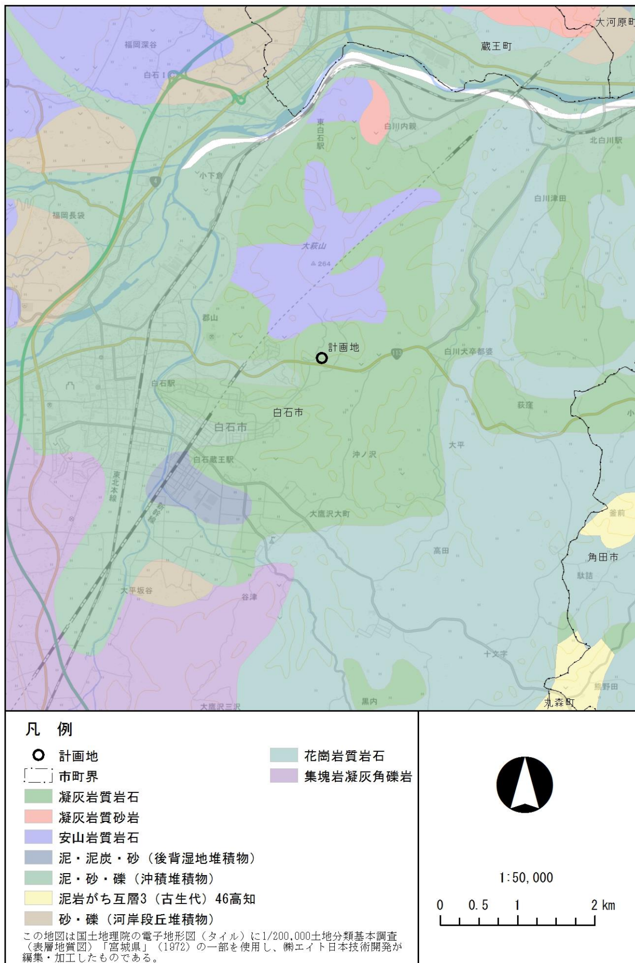
図 2-2-1 計画地周辺の地質
