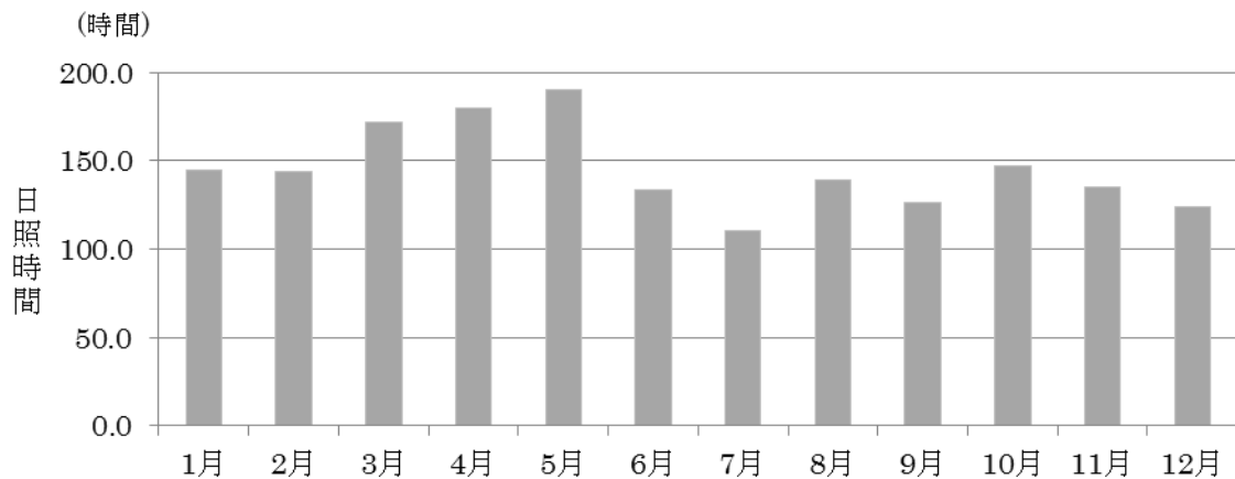
図 2-2-7 白石局における日照時間の推移
