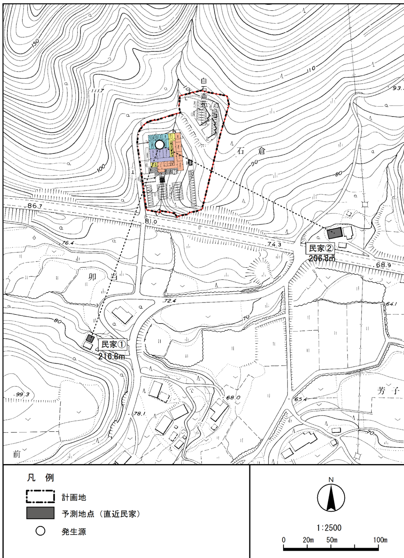
図 5-1-2 設備の配置位置及び騒音予測定点
