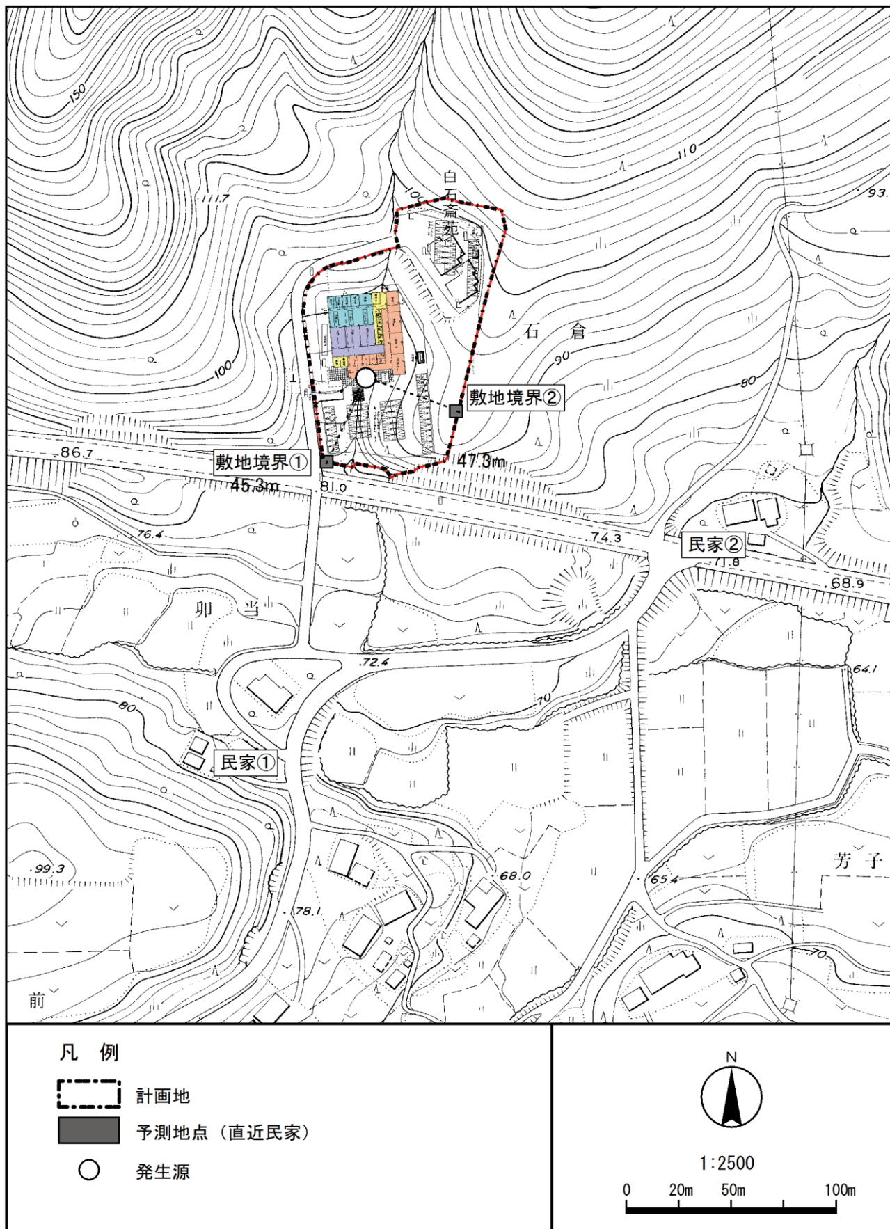
図 5- 1-1 建設機械配置位置及び騒音予測定点
