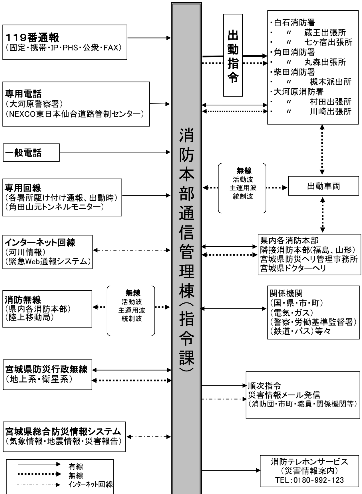
(1) 消防通信系統図
